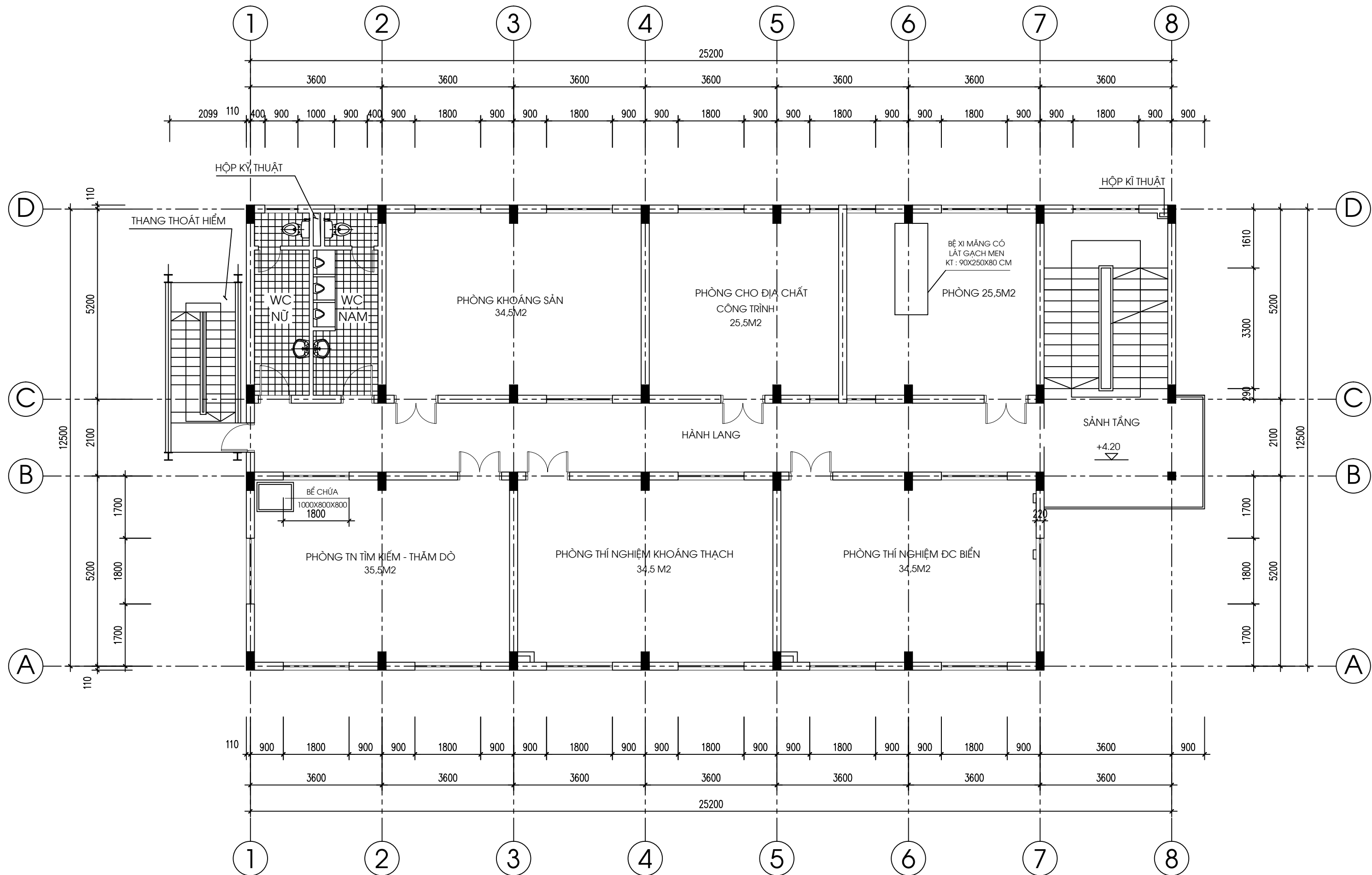
MẶT BẰNG TẦNG 4
