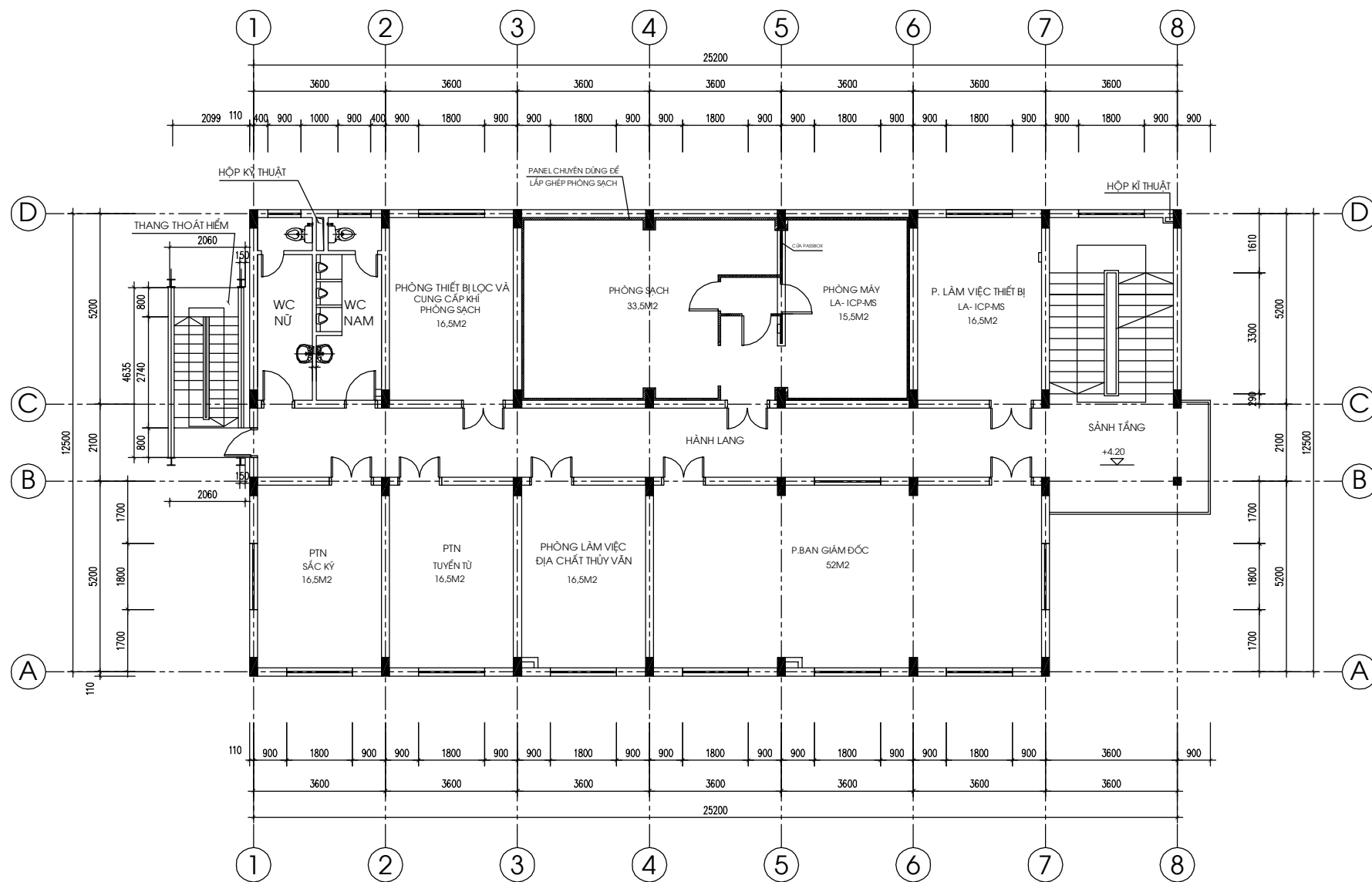
MẶT BẰNG TẦNG 2
