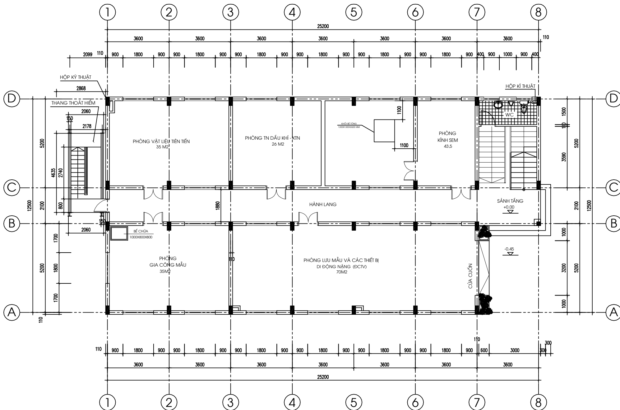
MẶT BẰNG TẦNG 1
