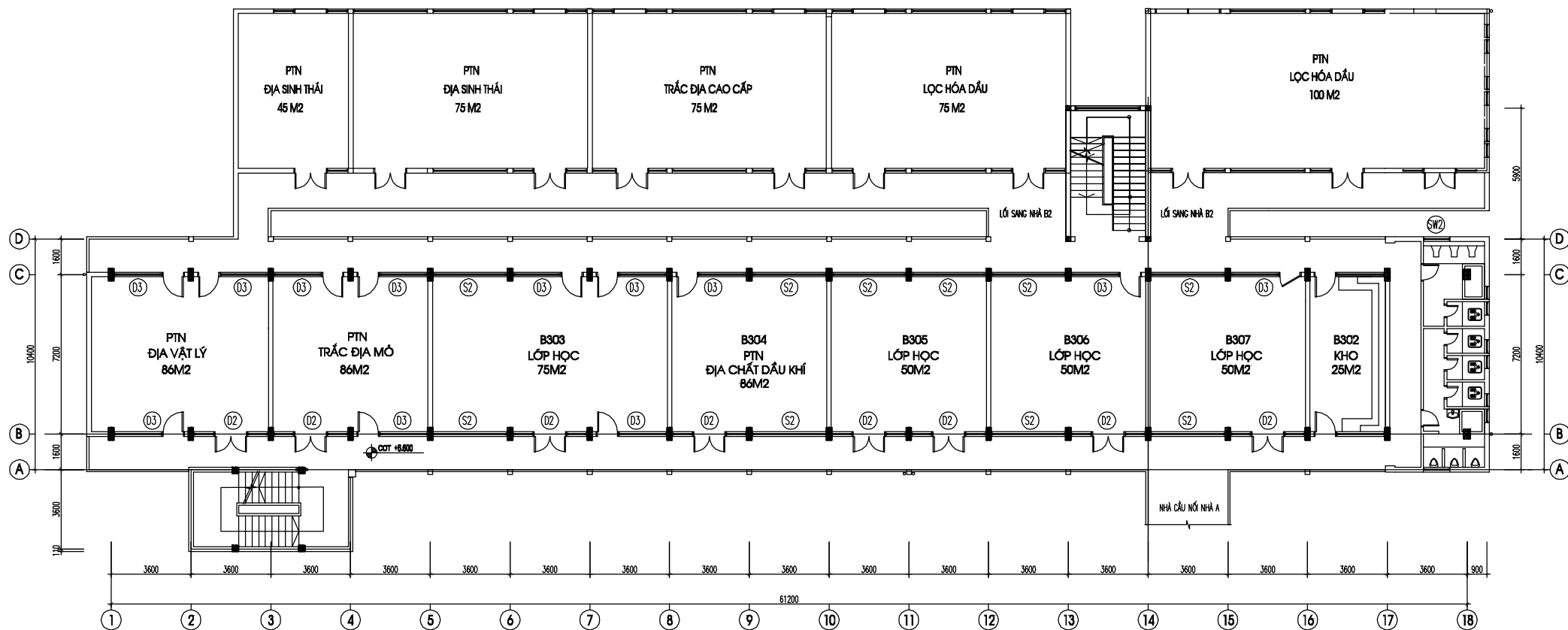
MẶT BẰNG TẦNG 3 NHÀ B
