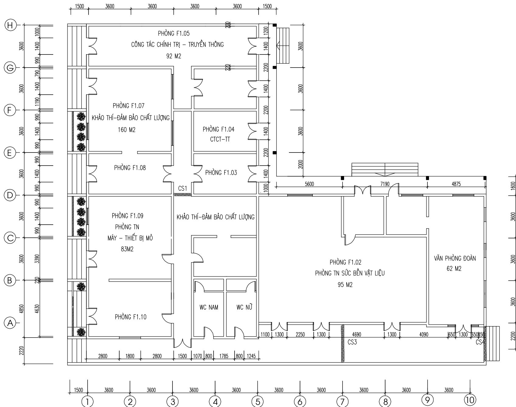
MẶT BẰNG TẦNG 1 NHÀ F
