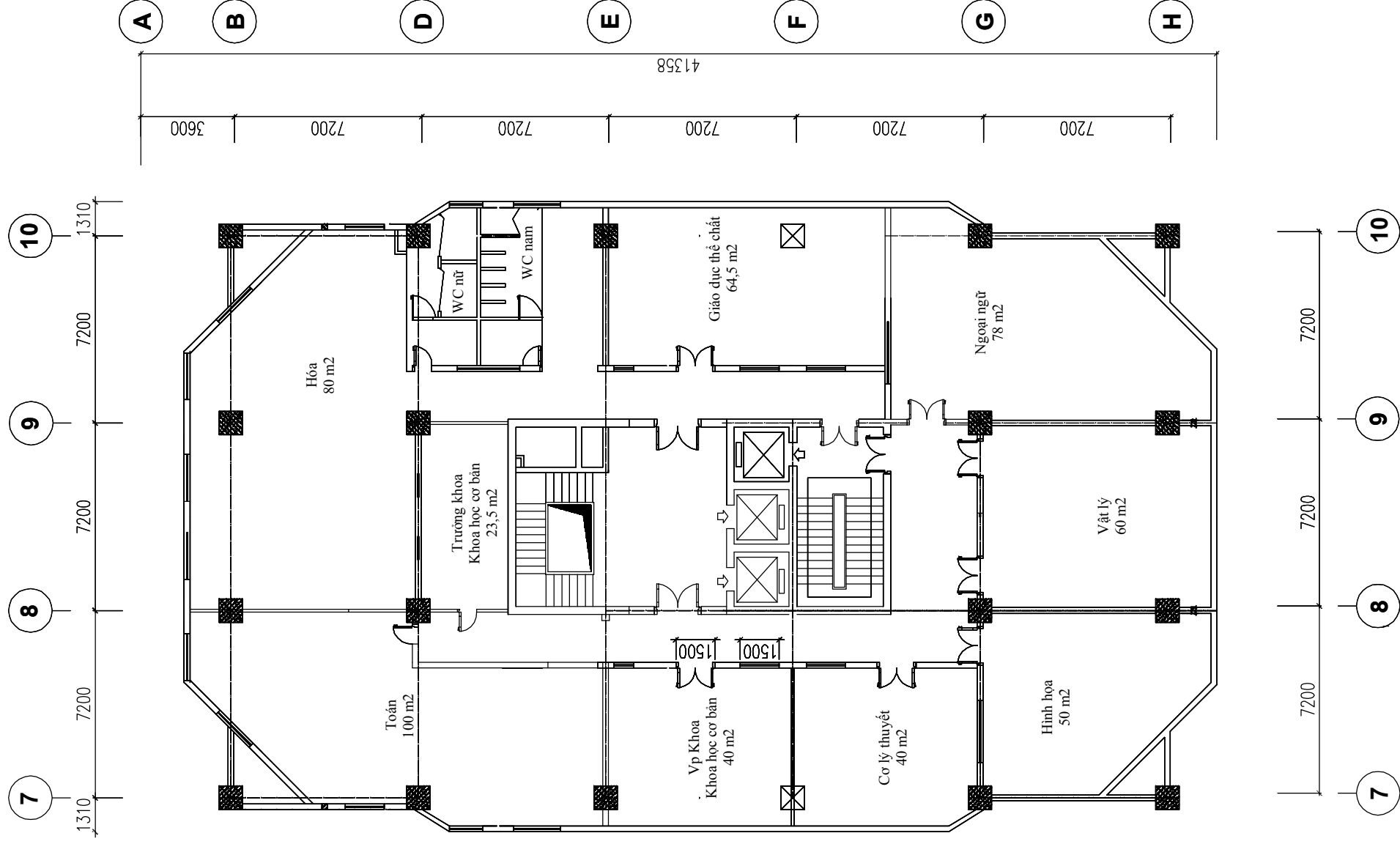
Mặt bằng tầng 11 nhà C12 tầng
