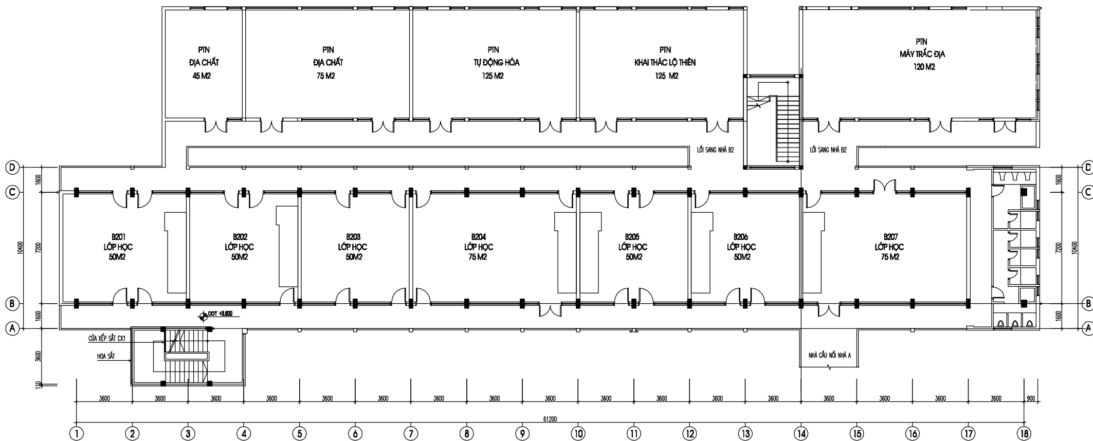
MẶT BẰNG TẦNG 2 NHÀ B
